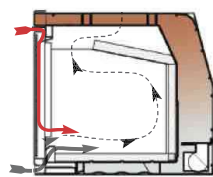
δευτερογενής αέρας αεροκουρτίνα
